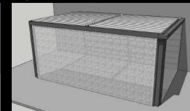
Store Zip en applique (coffre fixé contre les traverses à l'extérieur)
